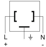
Zapojení konektoru
